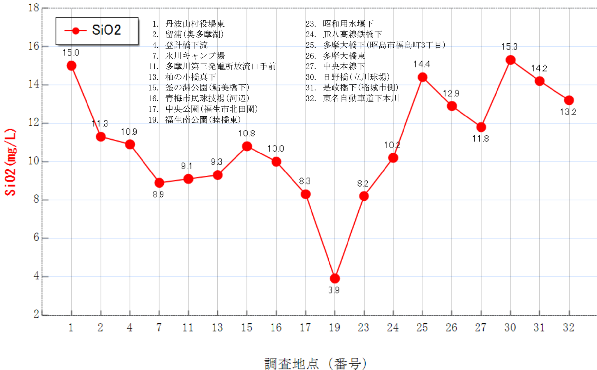
多摩川本川におけるSiO 2 の測定結果 (2022年6月5日)
