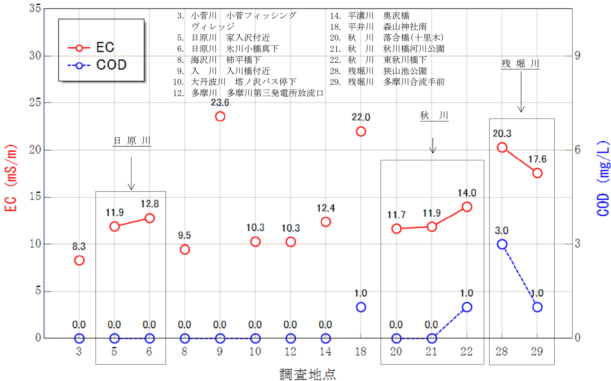
多摩川支川におけるEC・CODの測定結果(2022年6月5日)
