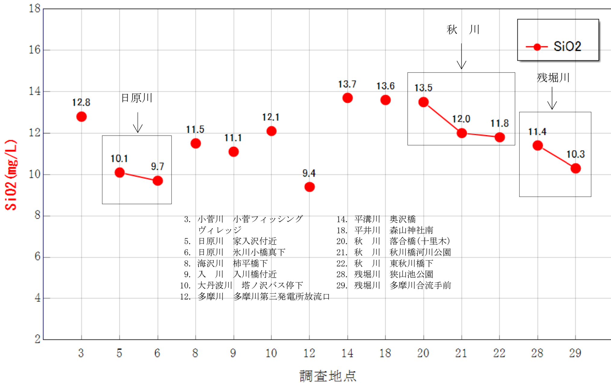
多摩川支川におけるSiO 2 の測定結果(2022年6月5日)
