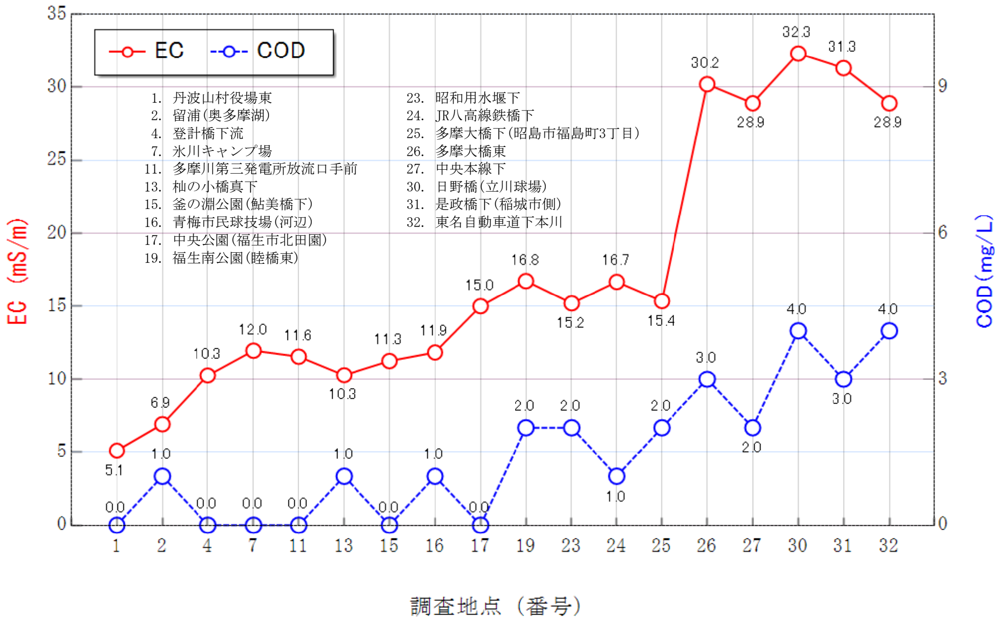
多摩川本川におけるEC・CODの測定結果(2022年6月5日)
