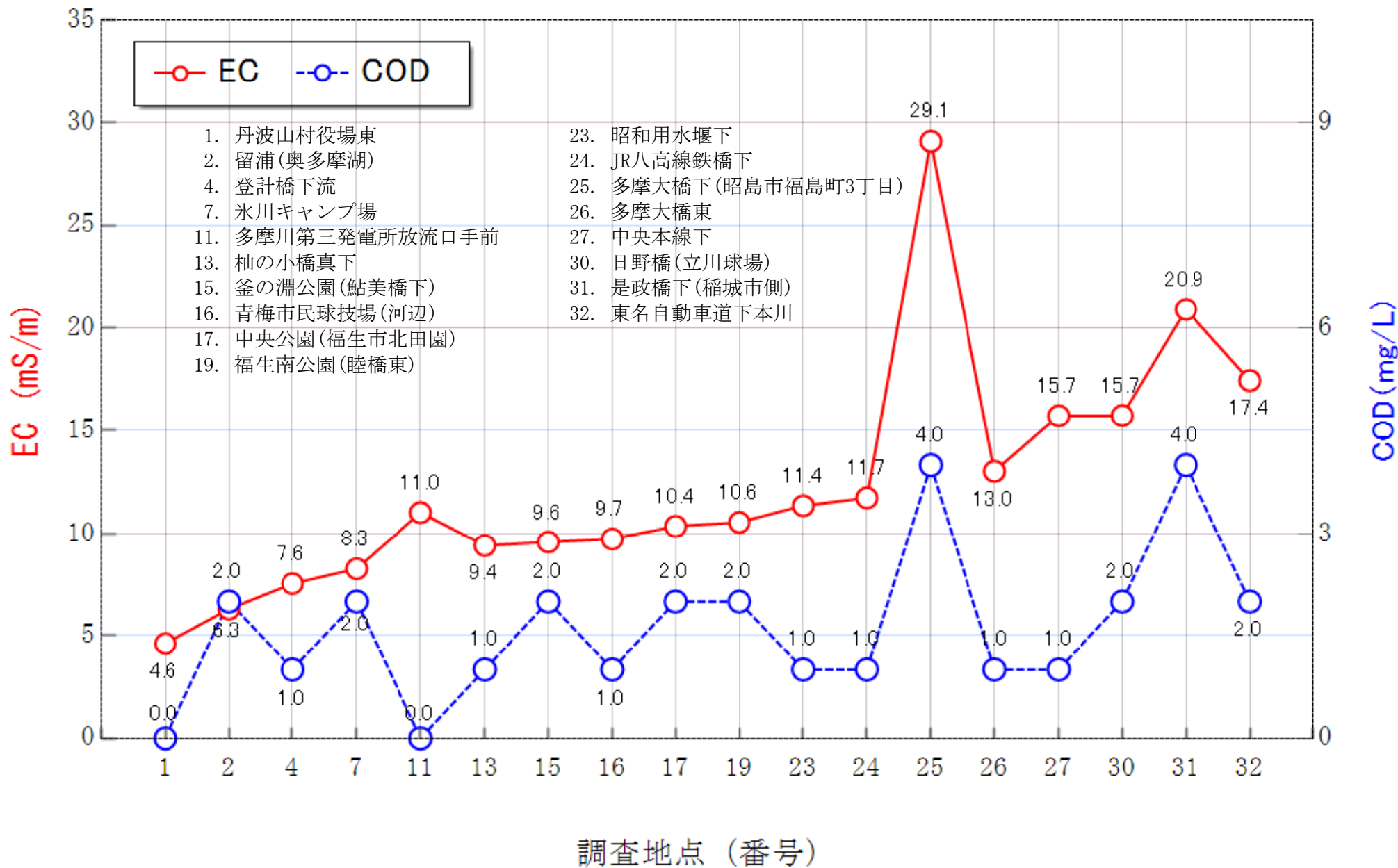
多摩川本川におけるEC・CODの測定結果(2023年6月10日)
