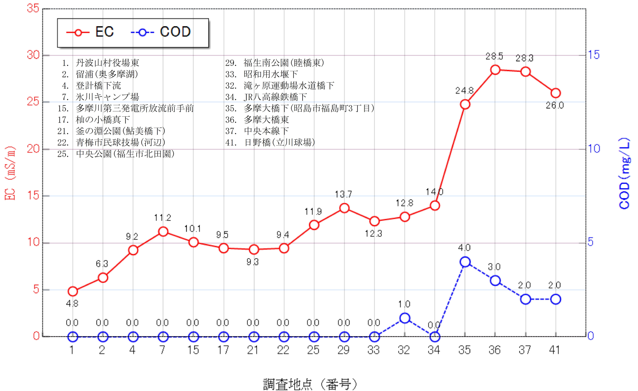
多摩川本川におけるEC・CODの測定結果(2020年8月17, 19, 21日)
