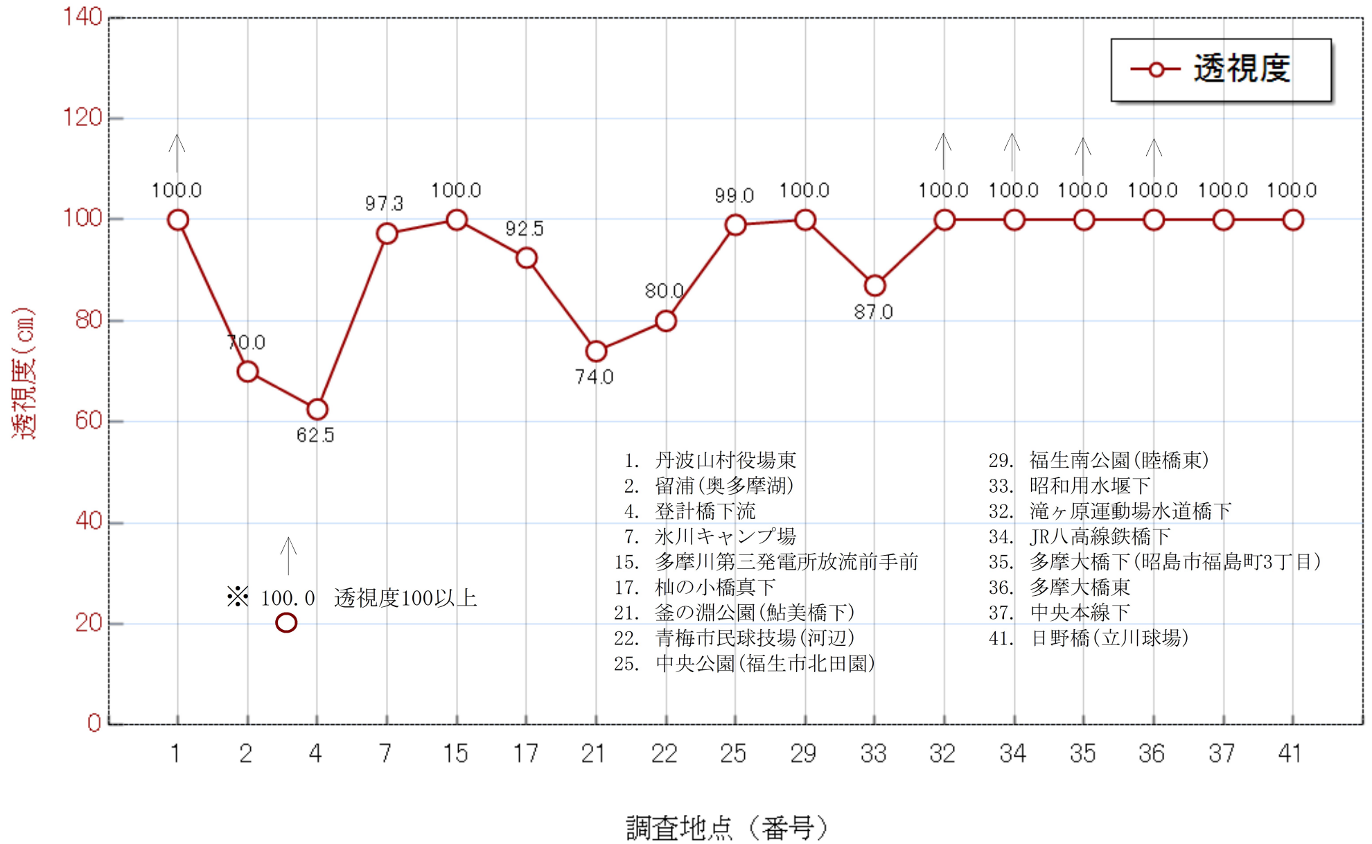
多摩川本川における透視度の測定結果(2020年8月17, 19, 21日)
